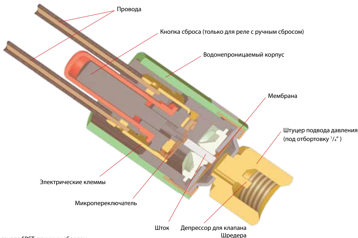
Рис. Контактная группа SPST с ручным сбросом
