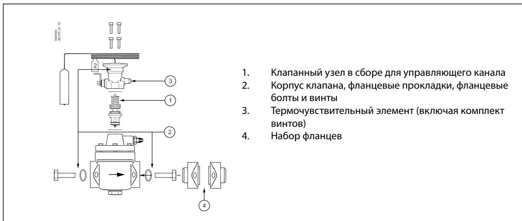
Клапан PHT 85 с фланцами под пайку или сварку
