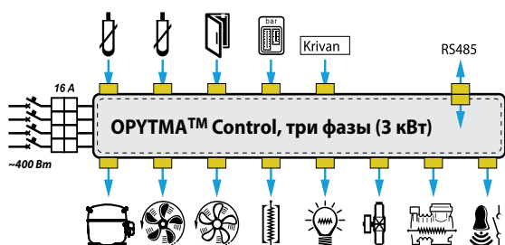
Optima™ Control, 3 фазы (3 кВт)
