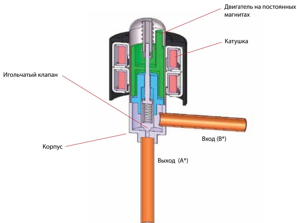
Чертеж поперечного сечения клапана серии ETS 6. * Показано для потока холодильного агента в режиме охлаждения
