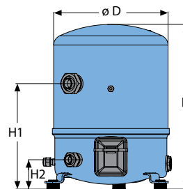
MT / MTZ / NTZ 2 цилиндра
