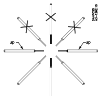
Установка датчика
