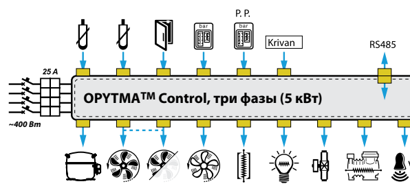
Optima™ Control, 3 фазы (5 кВт)
