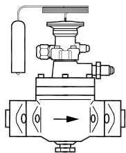
Клапан PHT 85 с фланцами под пайку или сварку
